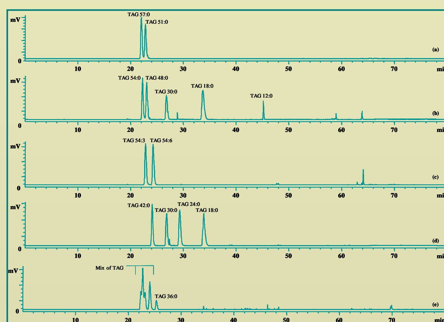
Fig. 2. HPLC-ELSD chromatograms for identification of TAG. TAG composition in figure (e): TAG 34:0 + TAG 54:3 + TAG 51:0 + TAG 48:0 + TAG 48:0 + TAG 48:0 + TAG 42:0 + TAG 36:0.
