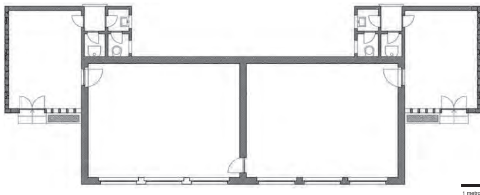
Planta da escola das Agras com a abertura interna entre as salas de aula.
