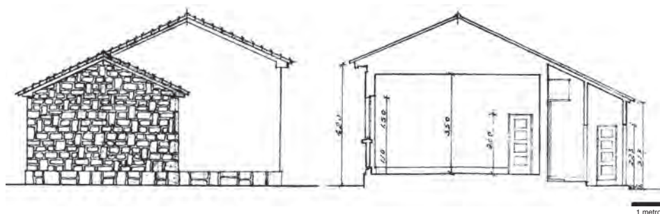
Desenhos originais do alçado lateral da escola da Serra da Vila (à esquerda) e corte (à direita).
