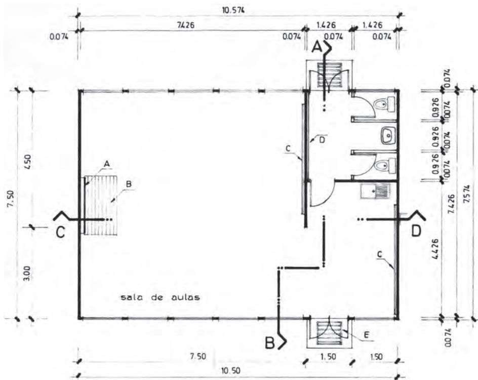
Desenho original da planta do pré-fabricado (Telescola).
