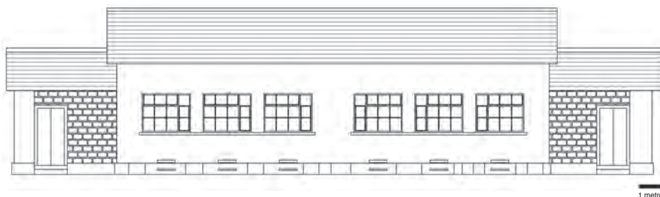
Alçado principal da escola das Agrads com os rasgos nas pedras do embasamento da parede.
